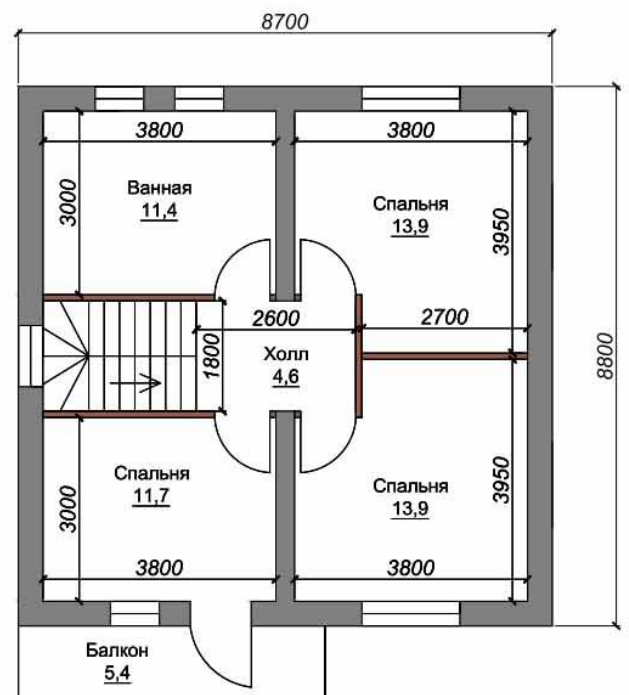
ПЛАН 2 ЭТАЖА
