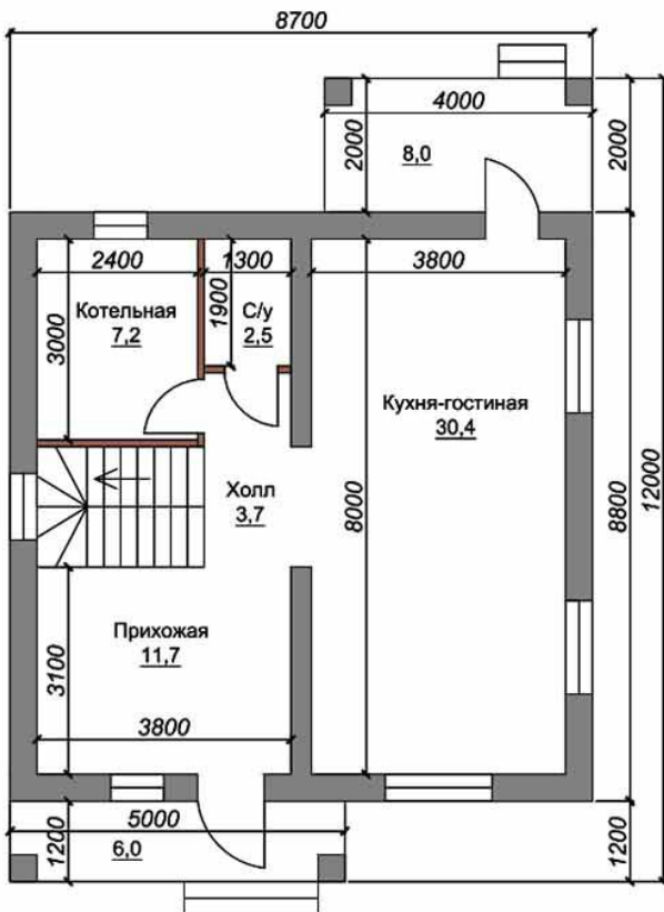
ПЛАН 1 ЭТАЖА
