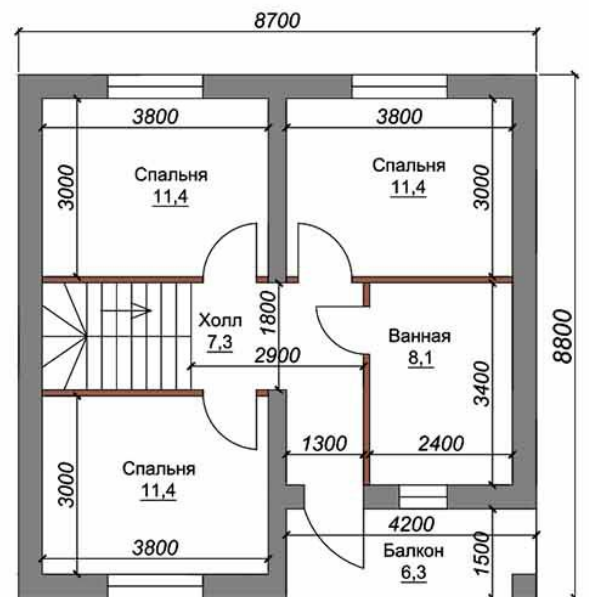
ПЛАН 2 ЭТАЖА
