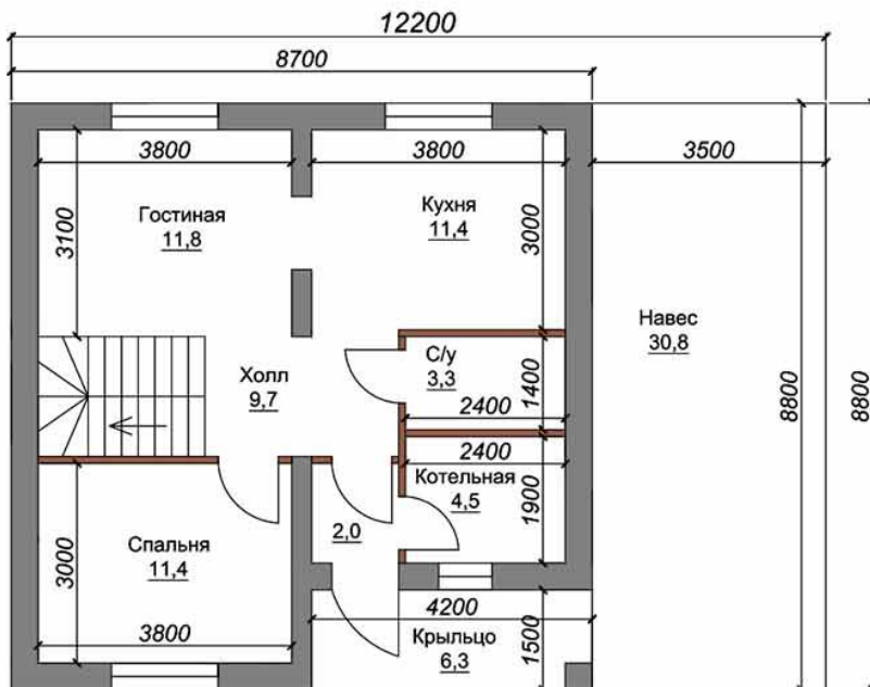
ПЛАН 1 ЭТАЖА
